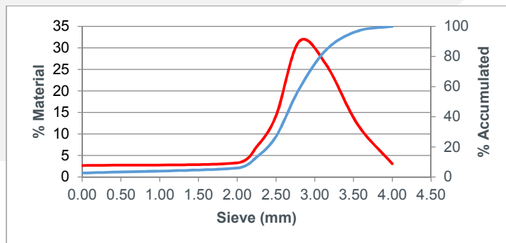
Granulometric Curve (CEN TS 14243)
